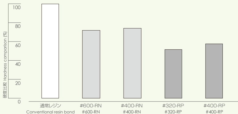
ボンド硬度比較(通常レジンボンドを100として) Hardness comparison (as conventional resin bond = 100)
