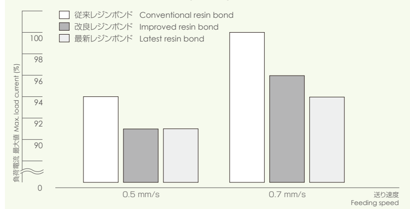
ネオジウム磁石 切断テスト時の負荷電流比較 (従来レジンボンド0.7mm/s時を100として) Load current comparison from the Neodymium magnet cutting test (as convention resin bond @ 0.7 mm/s = 100)
