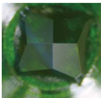
マイクロビッカース圧子先端の顕微鏡写真 Microphotograph of the micro-Vickers hardness-testing indenter's tip
