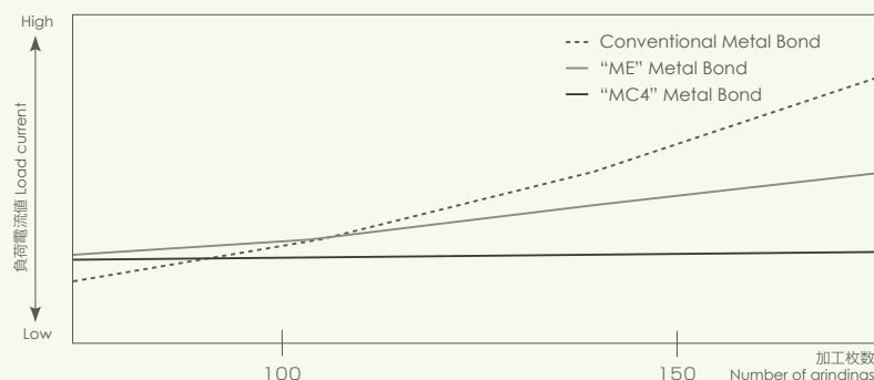
シリコンウェーハ加工テスト時の加工枚数による負荷電流の変化 Load current transition of grinding test of silicon wafer
