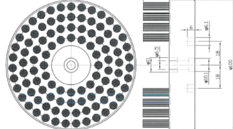
Ø100タイプ図
