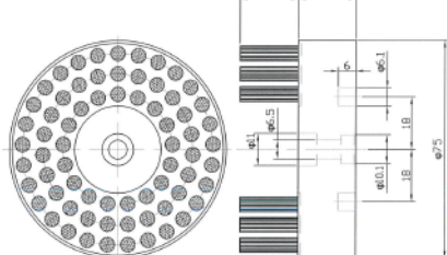
Ø75タイプ図
