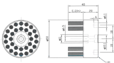
Ø50タイプ図
