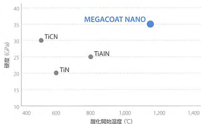
コーティング特性（耐摩耗性）
