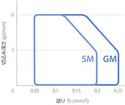
肩加工
