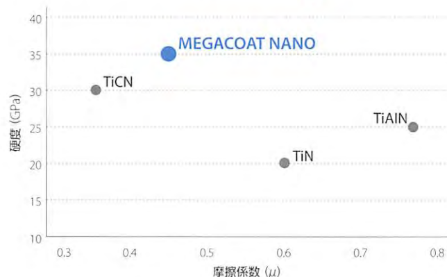
コーティング特性（耐溶着性）
