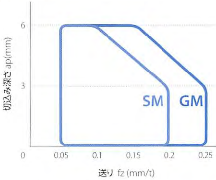
溝加工
