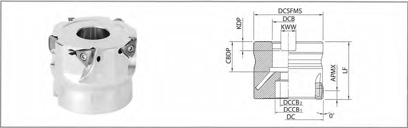
ホルダ寸法
