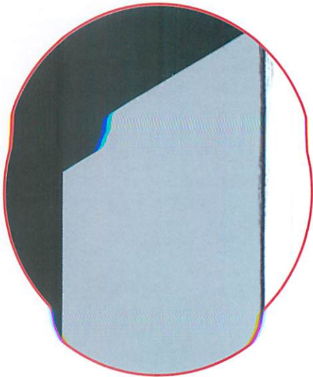
PCDドリルの刃部拡大写真(×30) ■ 高剛性設備の研削で鋭利な刃先を実現 ■ 刃部、外周部チップング8μm以下(写真製品)
