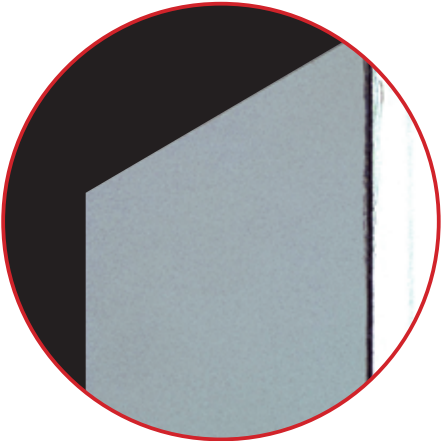
PCDドリルの刃部拡大写真(×30) ■ 高剛性設備の研削で鋭利な刃先を実現 ■ 刃部、外周部チップング8μm以下(写真製品)
